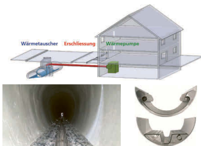
Kanalisation mit eingebautem Wärmetauscher
